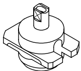
1011C1-19070 PICK-UP NOZZLE (MELF) (ID = \phi 0.9, OD = \phi 2.0) KME, CM92-MT
